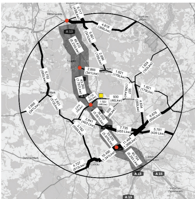
Tropical Islands Resort: Verkehrsbelastung im Nullfall
