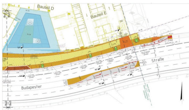
BIKINI BERLIN: Planung der Straßenbauflächen
