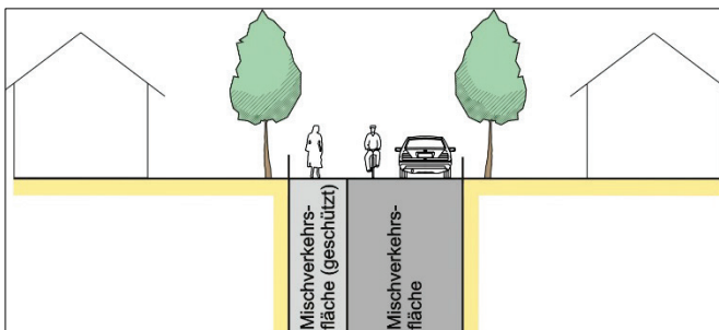
Pankow Erholungsanlagen: Prognostizierte Verkehrsmenge in der Spitzenstunde in Blankenburg, Netzhierarchie in Schildow-Waldeck und möglicher Ausbauquerschnitt für eine Wohnstraße
